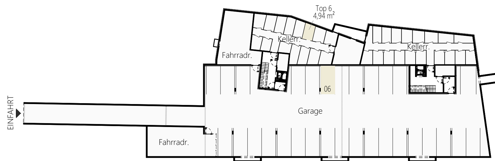
Untergeschoß Maßstabslos
