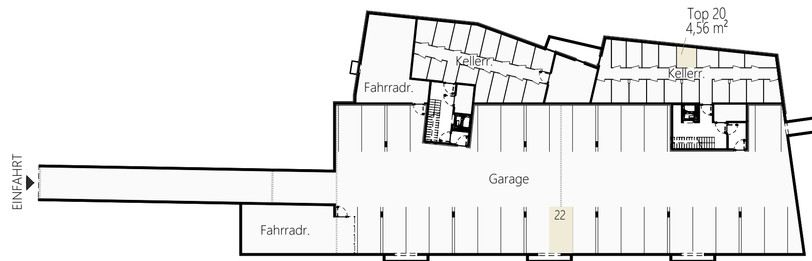
Untergeschoß Maßstabslos
