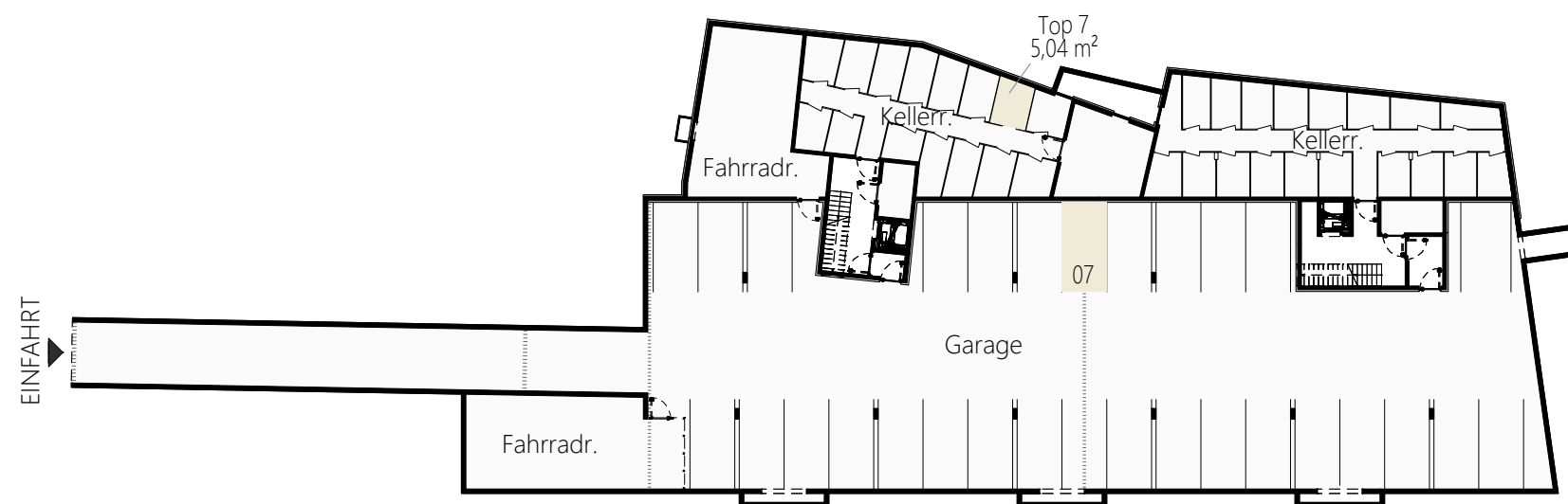
Untergeschoß Maßstabslos
