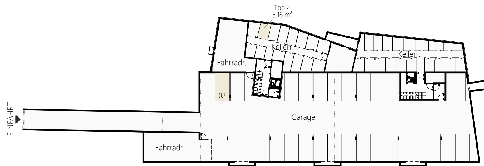
Untergeschoß Maßstabslos
