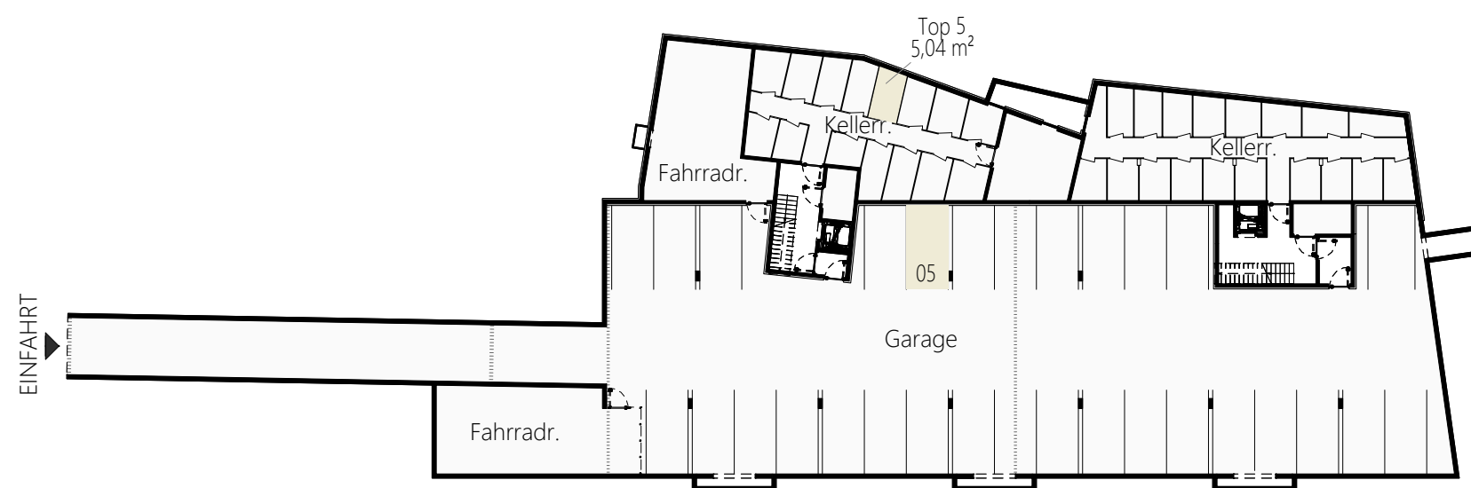
Untergeschoß Maßstabslos
