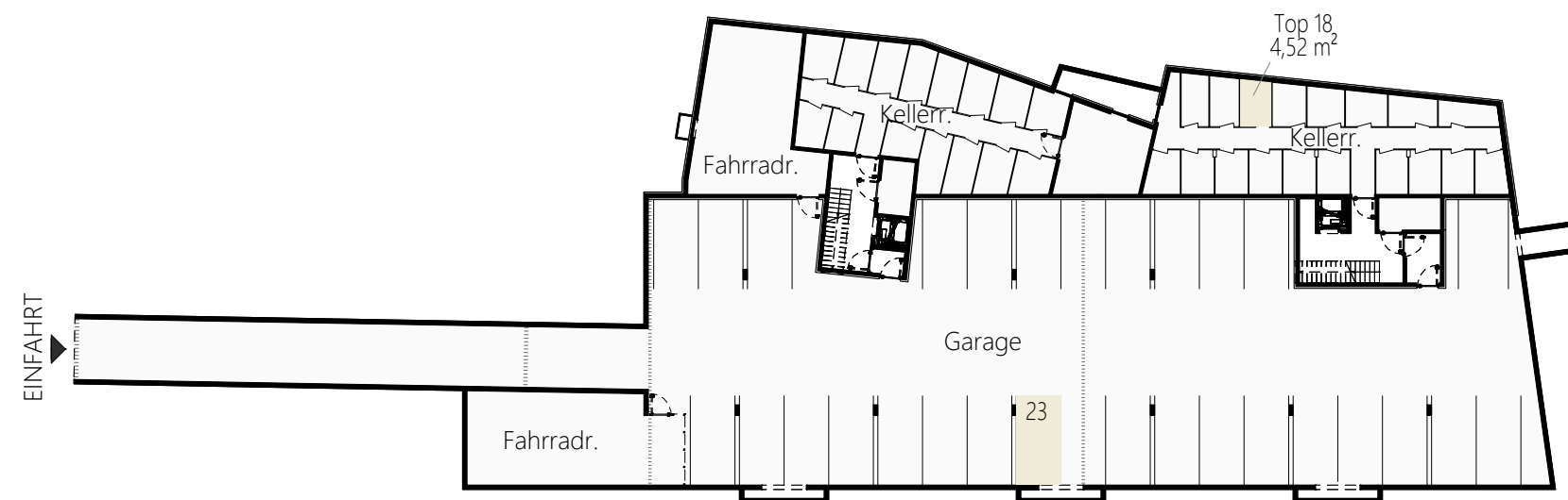
Untergeschoß Maßstabslos
